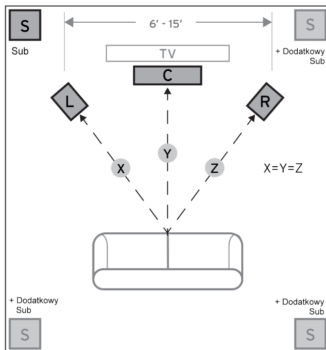
Rysunek 1 Rozstawienie głośników w miejscu odstuchu
