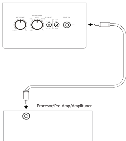
Wyjście LFE na Procesorze/Pre-Amp/Amplitunerze podłącz do wejścia LFE na wzmacniaczu subwoofera.
